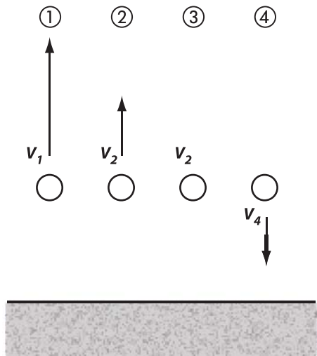
Fig. 5 - Balle lancée en l'air vue à quatre moments différents (les flèches représentent la grandeur et la direction de la vitesse V ).
