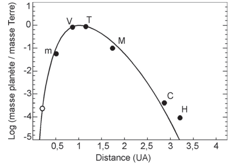
Figure 9. Comparaison entre les masses observées des planètes du système solaire interne et les prédictions du modèle hiérarchique (C et H correspondent aux pics en masse de la ceinture d'astéroïdes). L'éventuelle planète intramercurielle en n = 2 devrait avoir, si elle a pu résister aux perturbations et aux conditions que sa faible distance au soleil implique, une masse comprise entre 10^{-3} et 10^{-4} masse terrestre.
