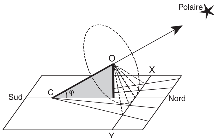
Fig. 7 - Passage du cadran équatorial au cadran horizontal
