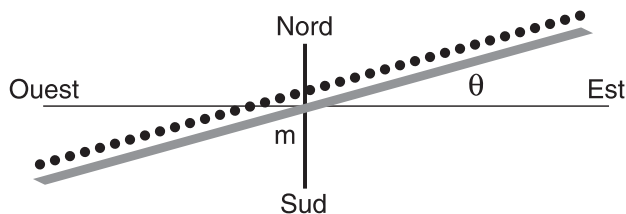
Fig. 12 - Détermination de la déclinaison du mur
