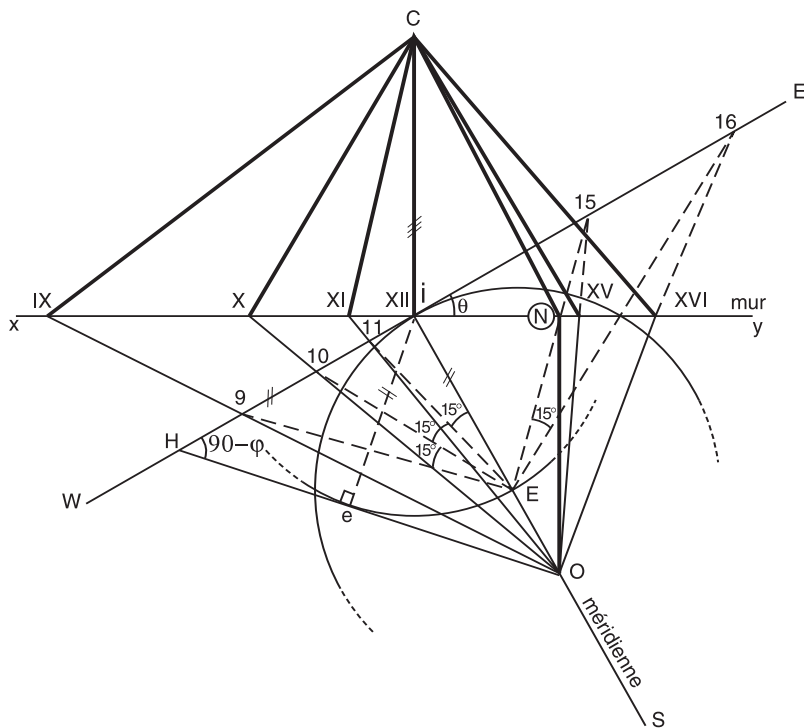
Fig. 14 - Tracé du cadran vertical-déclinant
